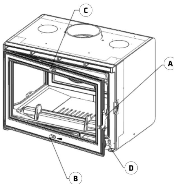
Figure n°9 - Éléments de fonctionnement de l'appareil
