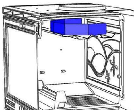
Figure n°11 - Deuxième déflecteur.
