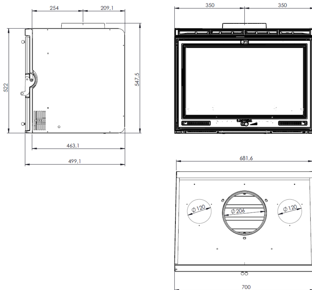
Figure n°1 - Dimensions en mm de l'appareil MIDI-700
