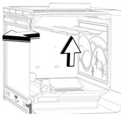
Figure n°10 - Vue de section avec le déflecteur principal placé
