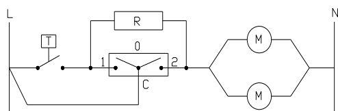
Figure n°12 - Schéma électrique des ventilateurs
