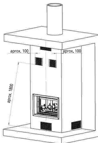
Figure n°4 - Schéma extérieur de la fermeture
