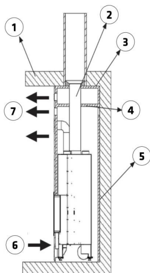
Figure n°3 - Schéma intérieur de la fermeture
