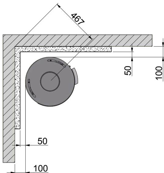
Installation en angle à 45°
