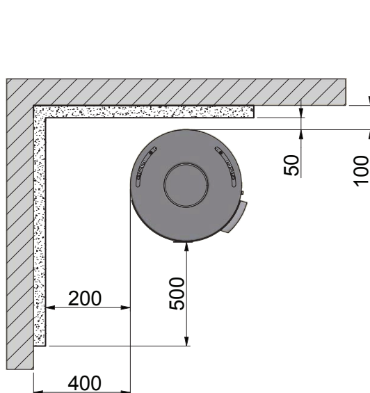
Installation parallèle contre le mur arrière
