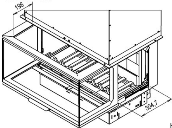
Ouverture tiroir
