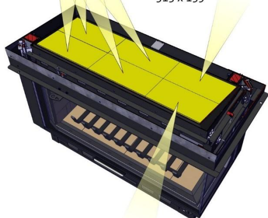
83168 Déflecteur inférieur latéral avant 309 x 159
