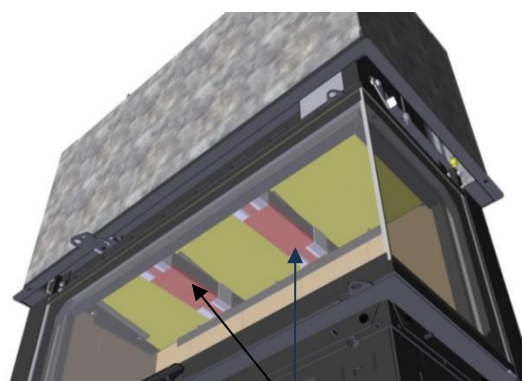
Boucliers thermiques maintenus par 4 brides chacun
